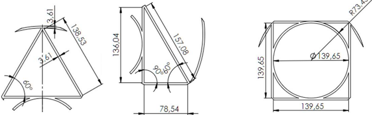
Detail A.
